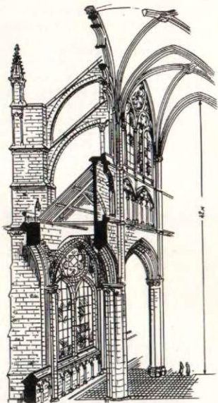
89. Схема конструкции собора в Амьене
